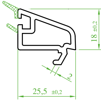
(ST 7450) “SÜRMETEC” Yapıştırma Contalı Tek Cam Çıtası “SURMETEC” Single Glazing Bead “SURMETEC” Приклеивающийся штапик с уплотнителем для одинарного стекла ماسکه زجاج (مفرد) مع فتيل لاصق
