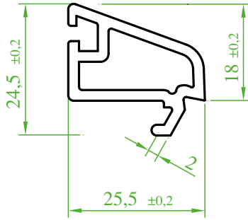
(ST 7510) “SÜRMETEC” Tek Cam Çıtası “SURMETEC” Single Glazing Bead “SURMETEC” Штапик для одинарного стекла ماسکه زجاج (مفرد)
