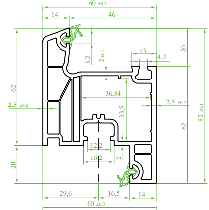
(ST 8310) "MEGATEC" Kanat Profili (Contalı) Sash Profile (Seal) Профиль створки (с уплотнителем) بروفیل الصترفه (مع الفتیل)
