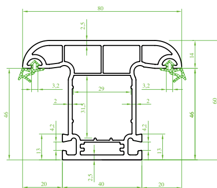
(ST 4210) “SOLOTEC” Orta kayıt Profili (Contalı) Mullion profile (Seal) Профиль импоста (с уплотнителем) بروفیل المنصف الثابت (مع الفیتل)
