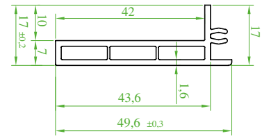
(ST 7700) "SÜRMETEC" Pervaz Profili Sill Joint Extension Profile Карнизный профиль بروفیل البرواز
