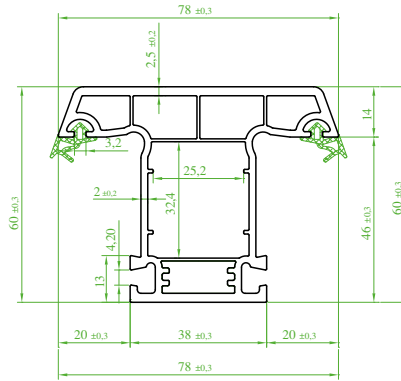
(ST 6122) "SÜPERTEC" Yeni Orta Kayıt Profili (Contalı) New Mullion Profile (Seal) Профиль импоста, новый (с уплотнителем) بروفیل المنصف الثابت جدید (مع الفتل)
