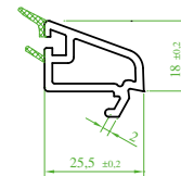
(ST 7450) "SÜRMETEC" Yap. Con. Tek Cam Çıtası Single Glazing Bead Приклеивающийся штапик с уплотнителем для одинарного стекла ماسكه زجاج (مفرد) مع قفیل لاصق
