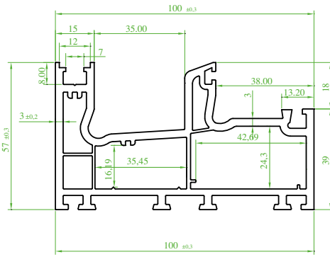
(ST 7340) "SÜRMETEC" Yeni Kasa Profili New Sliding Frame Profile Профиль коробки, новый بروفیل صندوق جدید
