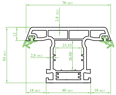
(ST 7410) "SÜRMETEC" Orta Kayıt Profili (Contalı) Mullion Profile (Seal) Профиль импоста (с уплотнителем) بروفیل المنصف الثابت (مع الفتیل)
