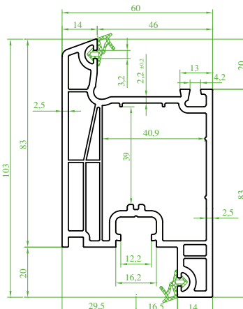
(ST 8410) "MEGATEC" Kapı Kanat Profili (Contalı) Door Sash Profile (Seal) Профиль дверного полотна (с уплотнителем) بروفیل صترفه باب (مع الفتیل)
