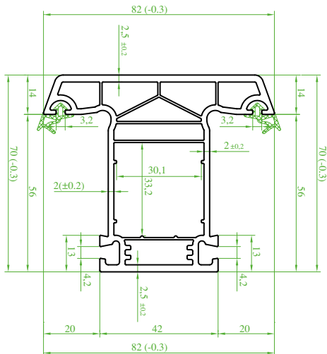
(ST 7122) "ULTRATEC" Eko. Orta Kayıt Profili (Contalı) Eco. Mullion Profile (Seal) Эко. Профиль импоста (с уплотнителем) أكو بروفیل المنصف الثابت (مع الفیتیل)
