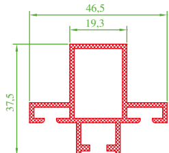
"SÜRMETEC" Alüminyum Karşılık Adaptörü Corresponding Adapter (Aluminum) Алюминиевый встречный адаптер وصله مقابل الألمنيوم
