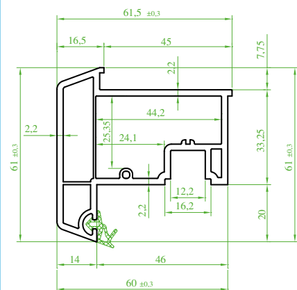
(ST 3310) “OVALTEC” Kanat Profili (Contalı) Sash Profile (Seal) Профиль створки (с уплотнителем) بروفیل الضرفه (مع الفیتل)
