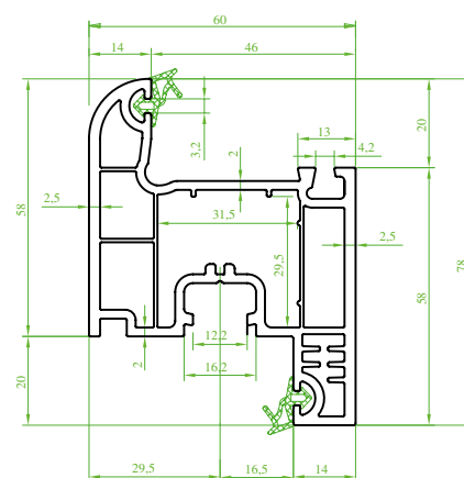
(ST 4310) “SOLOTEC” Kanat Profili (Contah) Sash Profile (Seal) Профиль створки (с уплотнителем) بروفيل الضرفه (مع الفتيل)
