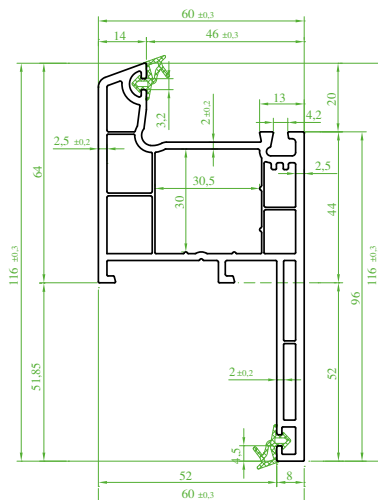
(ST 1410) “GROSSTEC” Pervazlı Kasa Profili (Contalı) Edge Frame Profile (Seal) Профиль коробки с карнизом (с уплотнителем) بروفیل الصندوق ذو البرواز (مع الفتیل)
