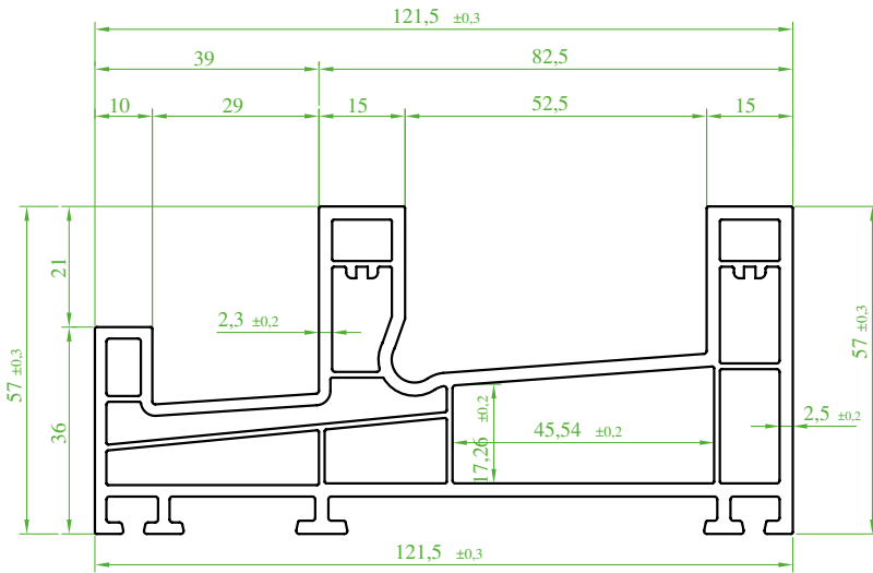
(ST 7600) "SÜRMETEC" Sineklikli Kasa Profili Swatter Frame Profile Профиль коробки с москитной сеткой بروفیل الصندوق (مانع الذباب)
