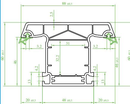
(ST 8810) "MEGATEC" Geniş Orta Kayıt Profili (Contalı) Wide Mullion Profile (Seal) Профиль импоста (с уплотнителем) بروفیل المنصف الثابت العريض (مع فتیل)
