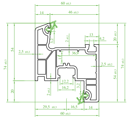
(ST 6133) "SÜPERTEC" Yeni Kanat Profili (Contalı) New Sash Profile (Seal) Профиль створки, новый (с уплотнителем) بروفیل الضرفه جدید (مع الفتل)
