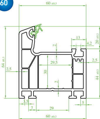
(ST 9110) "EXTRATEC" Kasa Profili (Contalı) Frame Profile (Seal) Профиль коробки (с уплотнителем) بروفیل الصندوق (مع فتل)
