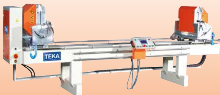
OCKK PVC / ALUMINIUM OTOMATİK ÇİFT KÖŞE KESİM MAKİNASI FULL AUTOMATIC DOUBLE MITRE SAW Автоматический Двухголовочный Станок Для Резки Профиля Из ПВХ
