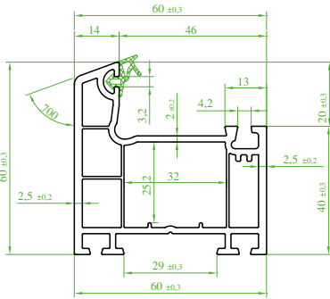
(ST 6111) "SÜPERTEC" Yeni Kasa Profili (Contalı) New Frame Profile (Seal) Профиль коробки, новый (с уплотнителем) بروفیل الصندوق جدید (مع فتل)
