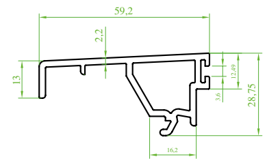
(ST 7370) "SÜRMETEC" Yeni Sabit Bölmeli Kasa Kapama Profili New Fixed Frame Closing Profile Закрытый Профиль коробки с фиксированными секциями بروفیل غطاء لتغطية صندوق ذو الأقسام الجديدة
