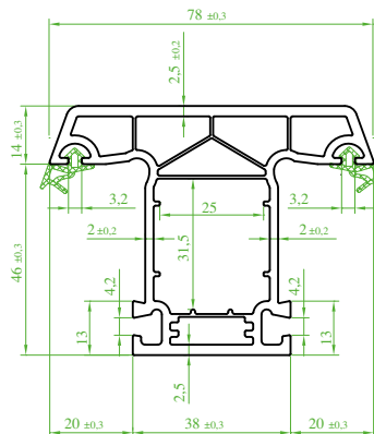
(ST 9210) "EXTRATEC" Orta kayıt Profili (Contalı) Mullion profile (Seal) Профиль импоста (с уплотнителем) بروفیل المنصف الثابت (مع الفتل)
