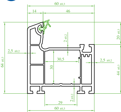
(ST1110) "GROSSTEC" Kasa Profili (Contalı) Frame Profile (Seal) Профиль коробки (с уплотнителем) بروفیل الصندوق (مع فتل)
