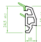
(ST 7460) "SÜRMETEC" Yap. Con. Çift Cam Çıtası Double Glass Lath with Adhesive Seal Приклеивающийся штапик с уплотнителем для двойного стекла ماسكه زجاج (مزدوج) مع قفیل لاصق
