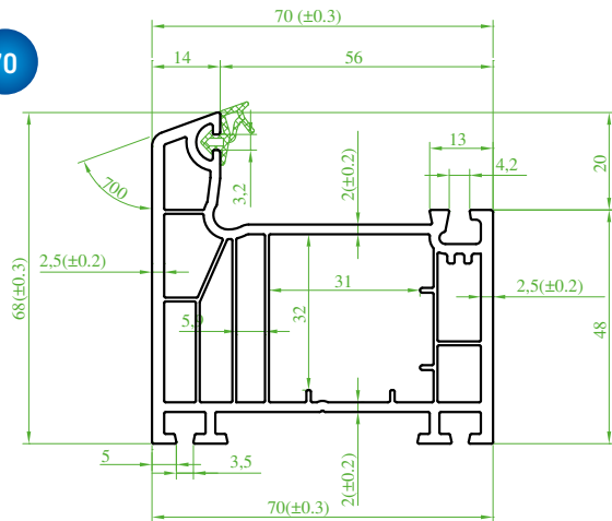
(ST 7121) "ULTRATEC" Eko. Kasa Profili (Contalı) Eco. Frame Profile (Seal) Эко. Профиль коробки (с уплотнителем) أكو بروفیل الصندوق (مع فیتیل)
