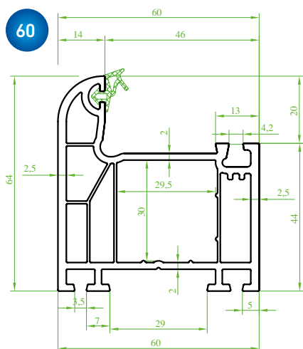
(ST 3110) "OVALTEC" Kasa Profili (Contali) Frame Profile (Seal) Профиль коробки (с уплотнителем) بروفيل الصندوق (مع فتل)
