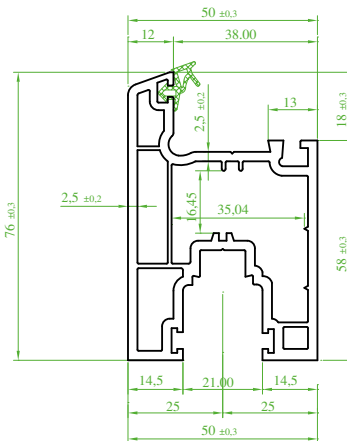
(ST 7310) "SÜRMETEC" Kanat Profili (Contalı) Sash Profile (Seal) Профиль створки (с уплотнителем) بروفیل الضرفه (مع الفتیل)
