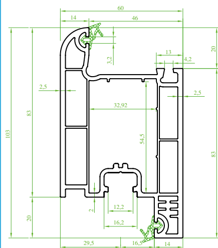
(ST 3410) "OVALTEC" Kapı Kanat Profili (Contali) Door Sash Profile (Seal) Профиль дверного полотна (с уплотнителем) بروفيل ضرفة باب (مع القليل)
