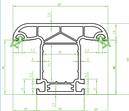
(ST 3210) "OVALTEC" Orta kayıt Profili (Contalı) Mullion profile (Seal) Профиль импоста (с уплотнителем) بروفیل المنصف الثابت (مع الفیتیل)
