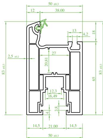
(ST 7330) "SÜRMETEC" Yeni Kanat Profili New Sliding Sash Profile Профиль створки, новый بروفیل الضرفه (جدید)
