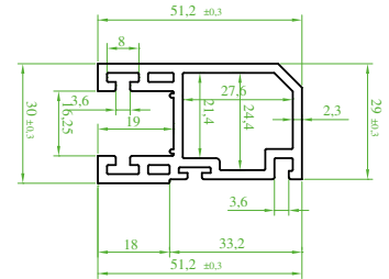
(ST 7800) "SÜRMETEC" Sineklikli Kanat Profili Swatter Sash Profile Профиль створки с москитной сеткой بروفیل الضرفه (مانع الذباب)
