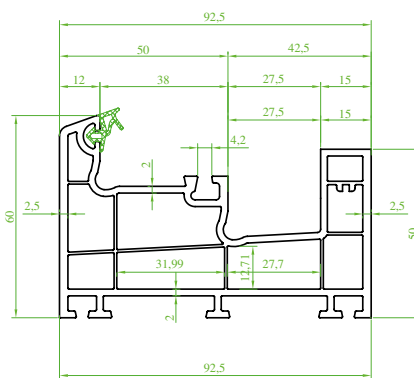
(ST 7360) "SÜRMETEC" Yeni Sabit Bölmeli Kasa Profili (Contalı) New Fixed Frame Slider (Seal) Профиль коробки с фиксированными секциями (с уплотнителем) بروفیل صندوق سحاب ذو أقسام ثابتة جدید (مع الفتیل)
