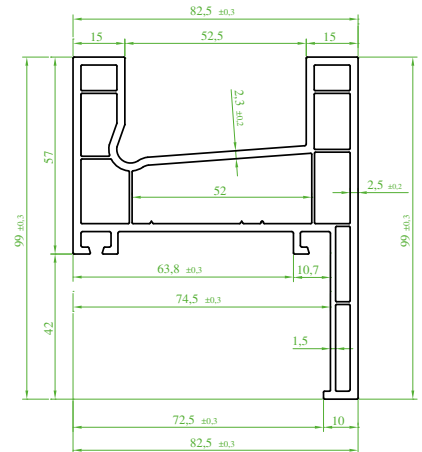
(ST 7900) "SÜRMETEC" Pervazlı Kasa Profili Edge Frame Profile Профиль коробки с карнизом بروفیل الصندوق ذو البرواز
