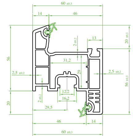
(ST 6133) "SÜPERTEC" Yeni Kanat Profili (Contalı) New Sash Profile (Seal) Профиль створки, новый (с уплотнителем) بروفیل الضرفه جدید (مع الفتل)
