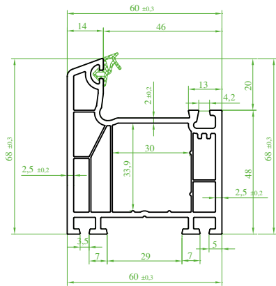
(ST 8110) "MEGATEC" Kasa Profili (Contalı) Frame Profile (Seal) Профиль коробки (с уплотнителем) بروفیل الصندوق (مع فتیل)
