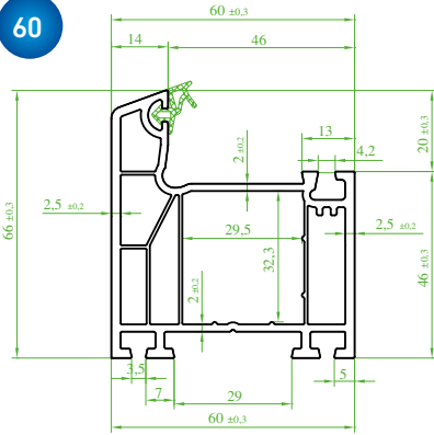
(ST 2110) "DIVATEC" Kasa Profili (Contalı) Frame Profile (Seal) Профиль коробки (с уплотнителем) بروفیل الصندوق (مع فتیل)
