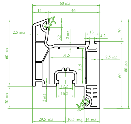
(ST 2310) "DIVATEC" Kanat Profili (Contalı) Sash Profile (Seal) Профиль створки (с уплотнителем) بروفیل الصترفه (مع الفتیل)
