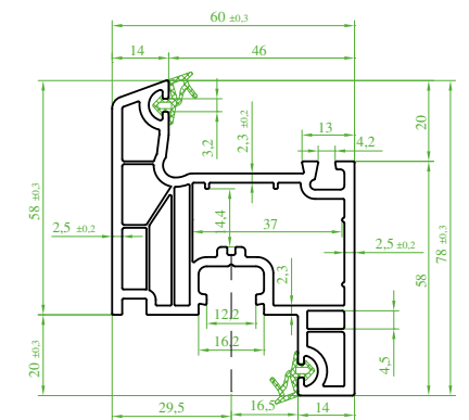
(ST 9310) "EXTRATEC" Kanat Profili (Contalı) Sash Profile (Seal) Профиль створки (с уплотнителем) بروفیل الضرفه (مع الفتل)
