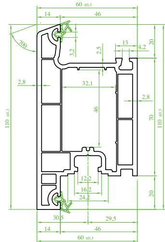
(ST 8460) "MEGATEC" Dışa Açılır Kapı Profili (Contalı) Outward Opening Door Sash Profile (Seal) Профиль двери открывающейся наружу (с уплотнителем) بروفیل باب یفتح للخارج (مع الفتیل)
