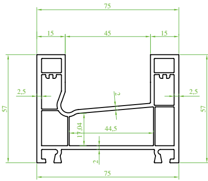
(ST 7340) "SÜRMETEC" Yeni Kasa Profili New Sliding Frame Profile Профиль коробки, новый بروفیل صندوق جدید
