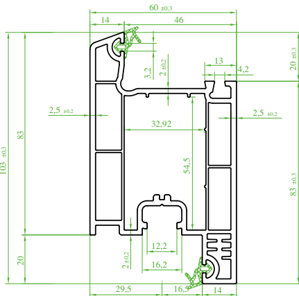
(ST 2410) "DIVATEC" Kapı Kanat Profili (Contalı) Door Sash Profile (Seal) Профиль дверного полотна (с уплотнителем) بروفیل صترفه باب (مع الفتیل)
