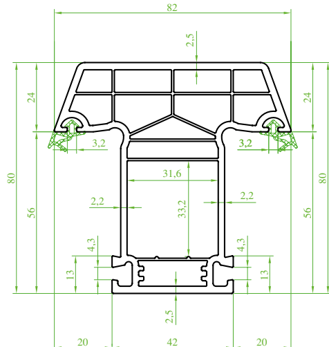
(ST 8030) ULTRAPLUS "80 X 70" Orta Kayıt Profili (Contalı) "80 X 70" Mullion Profile (Seal) "80 X 70" Профиль импоста (с уплотнителем) "80 X 70" بروفیل المنصف الثابت (مع الفیتیل)
