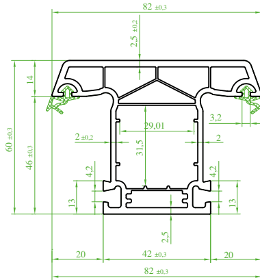
(ST 8210) "MEGATEC" Orta kayıt Profili (Contalı) Mullion profile (Seal) Профиль импоста (с уплотнителем) بروفیل المنصف الثابت (مع الفتیل)
