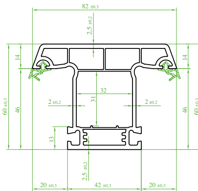
(ST 1210) "GROSSTEC" Orta kayıt Profili (Contalı) Mullion profile (Seal) Профиль импоста (с уплотнителем) بروفیل المنصف الثابت (مع الفتل)
