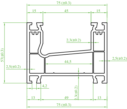
(ST 7120) "SÜRMETEC" Kayıtlı Kasa Profili Mullion Profile Профиль коробки с импостом بروفیل صندوق مع المنصف
