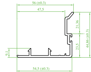
(ST 7210) "SÜRMETEC" Yeni Kilitleme Profili New Interlocking Profile Блокирующий профиль بروفیل الإقفال جدید
