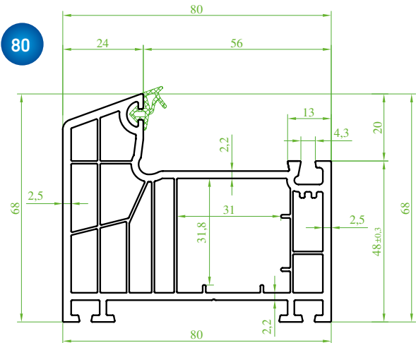
(ST 8010) ULTRAPLUS "80 X 70" Kasa Profili (Contalı) "80 X 70" Frame Profile (Seal) "80 X 70" Профиль коробки (с уплотнителем) "80 X 70" بروفیل الصندوق (مع فیتیل)
