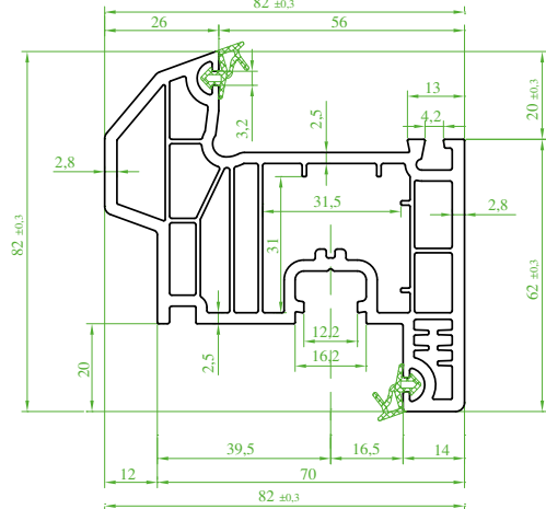
(ST 7013) "ULTRATEC" Damlalık Kanat Profili (Contalı) Self Drainage Sash Profile (Seal) Профиль створки с отводом конденсата (с уплотнителем) (ST 7013) بروفیل الضرفه (معقوس)
