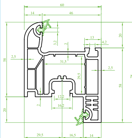
(ST 3310) “OVALTEC” Kanat Profili (Contalı) Sash Profile (Seal) Профиль створки (с уплотнителем) بروفیل الضرفه (مع الفیتل)
