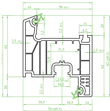
(ST 7123) "ULTRATEC" Eko. Kanat Profili (Contalı) Eco. Sash Profile (Seal) Эко. Профиль створки (с уплотнителем) أكو بروفیل الضرفه (مع الفیتیل)
