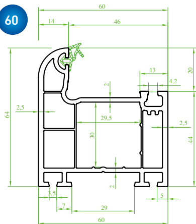
(ST 4110) “SOLOTEC” Kasa Profili (Contah) Frame Profile (Seal) Профиль коробки (с уплотнителем) بروفيل الصندوق (مع فتل)
